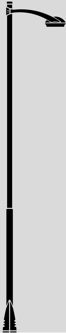
Saiph éclairage en tête avec bras h 6, 7, 8 e 9 m base Ø 36 x 50 cm produit d'éclairage Light 34
