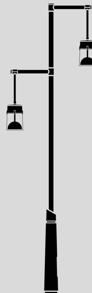
Chara éclairage en tête avec bras h 5, 6 et 7 m base Ø 27 cm
