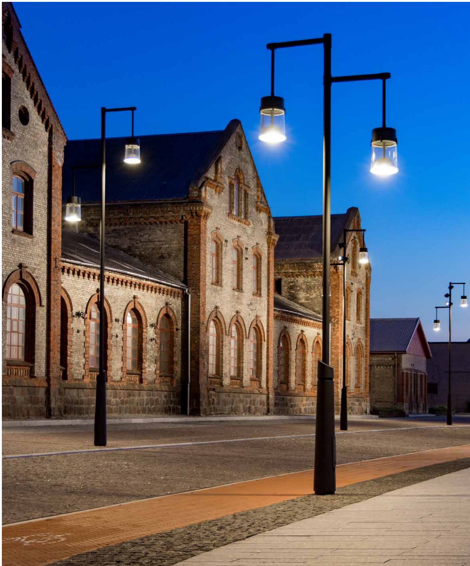
Chara éclairage en tête avec bras Bras à double départ h 5 e 7m
