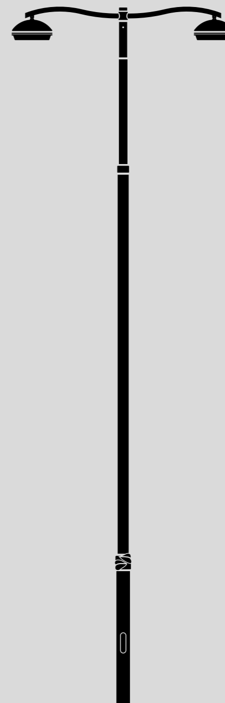
Propus éclairage en tête avec bras h 7, 8 et 9 m base Ø 16 et 17 cm produit d'éclairage Light 34
