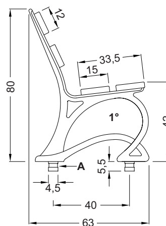
Fianco - sostegni Sx-Dx
