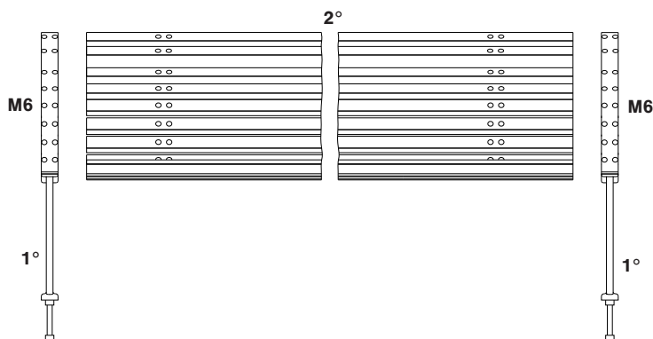
Vue éclatée
